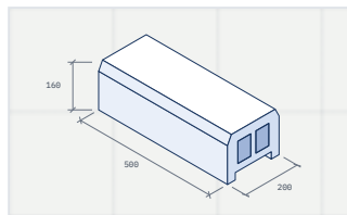
Hourdis de 16
